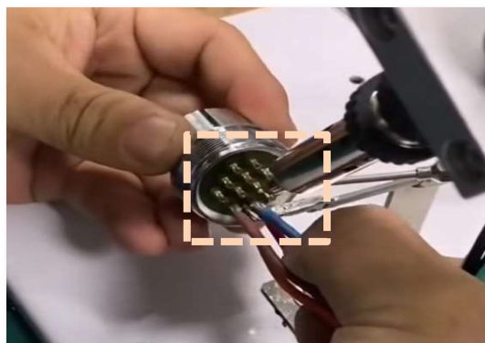
航空插头焊接
