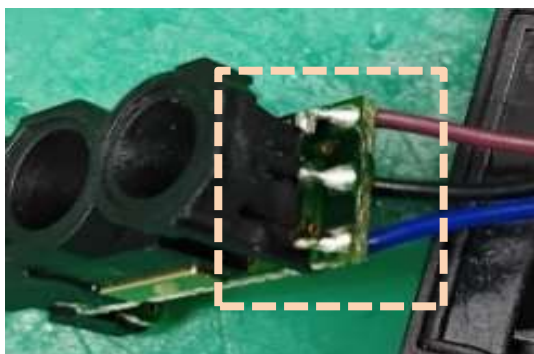
线材与基板焊接
