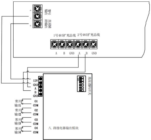
ACP3-RY08 8 路可编程继电器输出控制模块接线示意图
