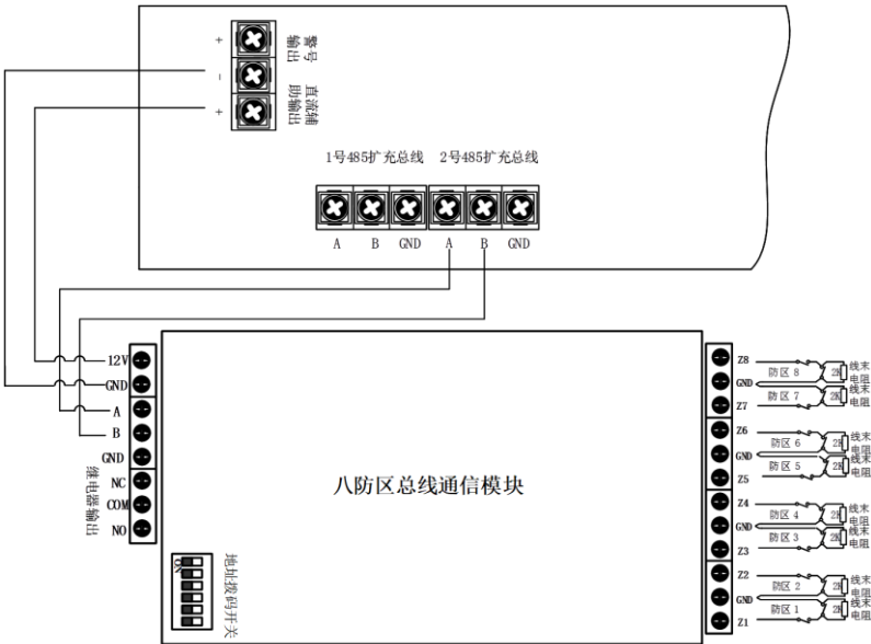
ACP3-DF08 8 防区总线通信模块接线示意图
