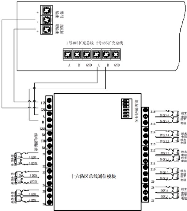
ACP3-DF16 16 防区总线通信模块接线示意图
