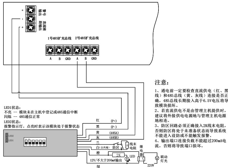
ACP3-DF01 单防区单输出总线通信模块接线示意图
