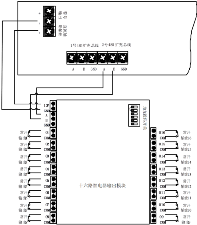
ACP3-RY16 16 路可编程继电器输出控制模块接线示意图
